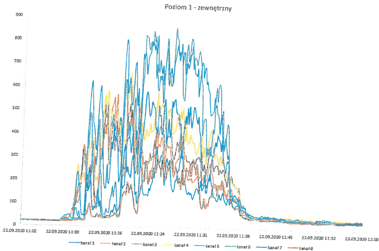
Fotografia 23. Wykres temperatury Poziom 1 - na zewnątrz
