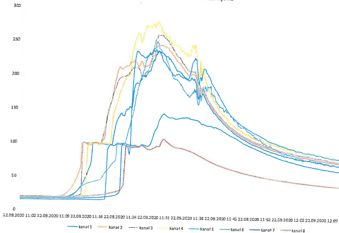
Fotografia 26. Wykres temperatury Poziom 2 - na styku warstwy zbrojącej z termoizolacją
