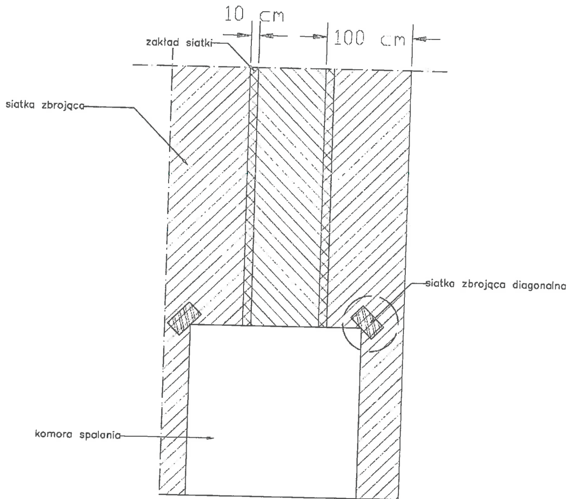
Fotografia 18. Ogólny schemat układu siatki zbrojącej
