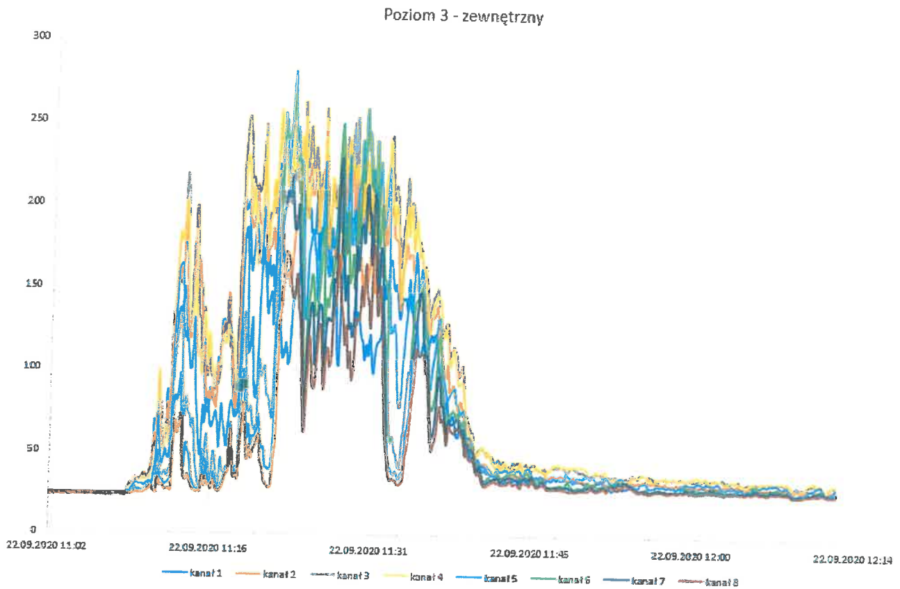
Fotografia 25. Wykres temperatury Poziom 3 - na zewnątrz Poziom 2 - warstwa zbrojona
