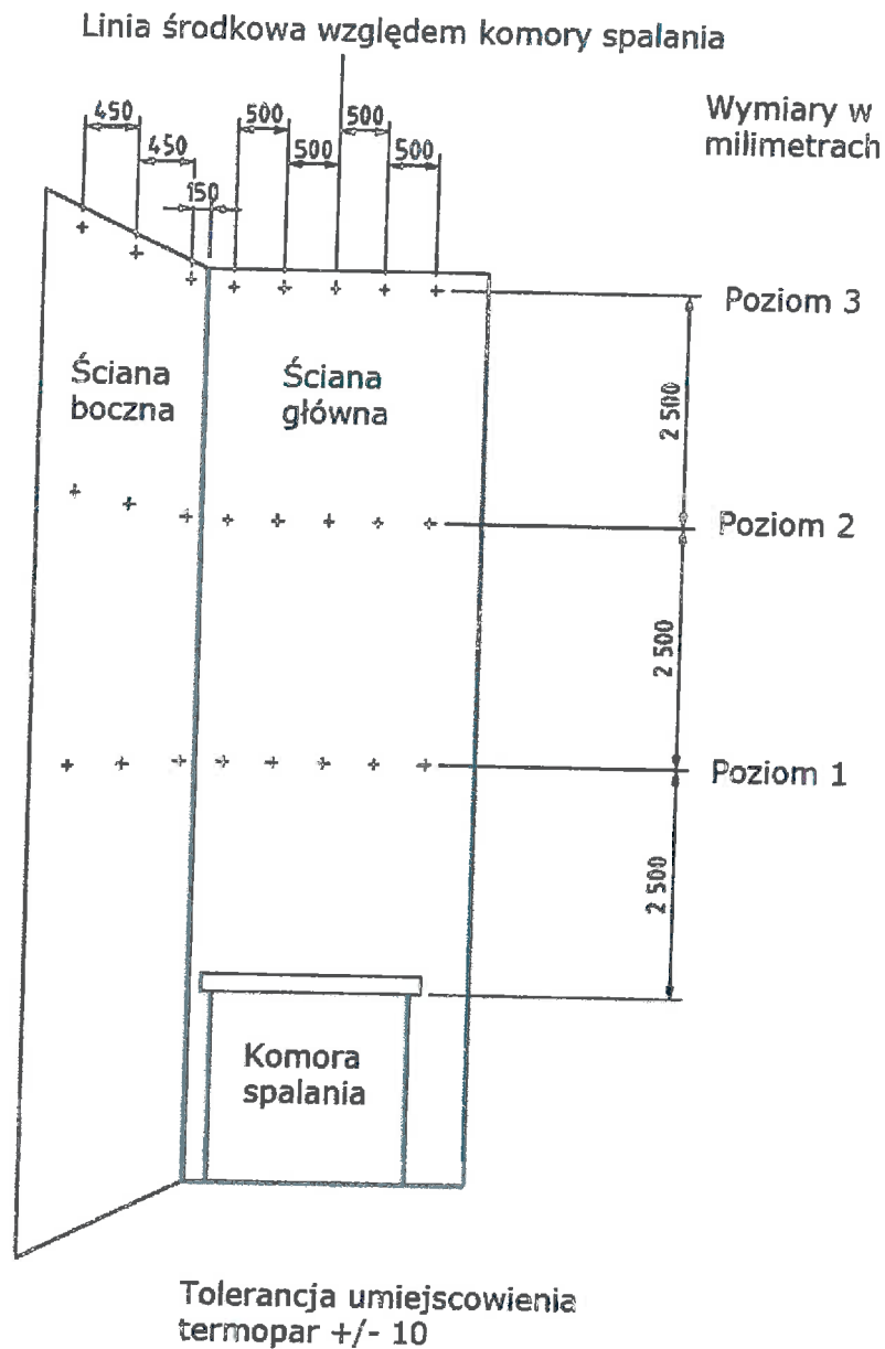
Fotografia 22. Schemat rozmieszczenia i identyfikacja termopar
