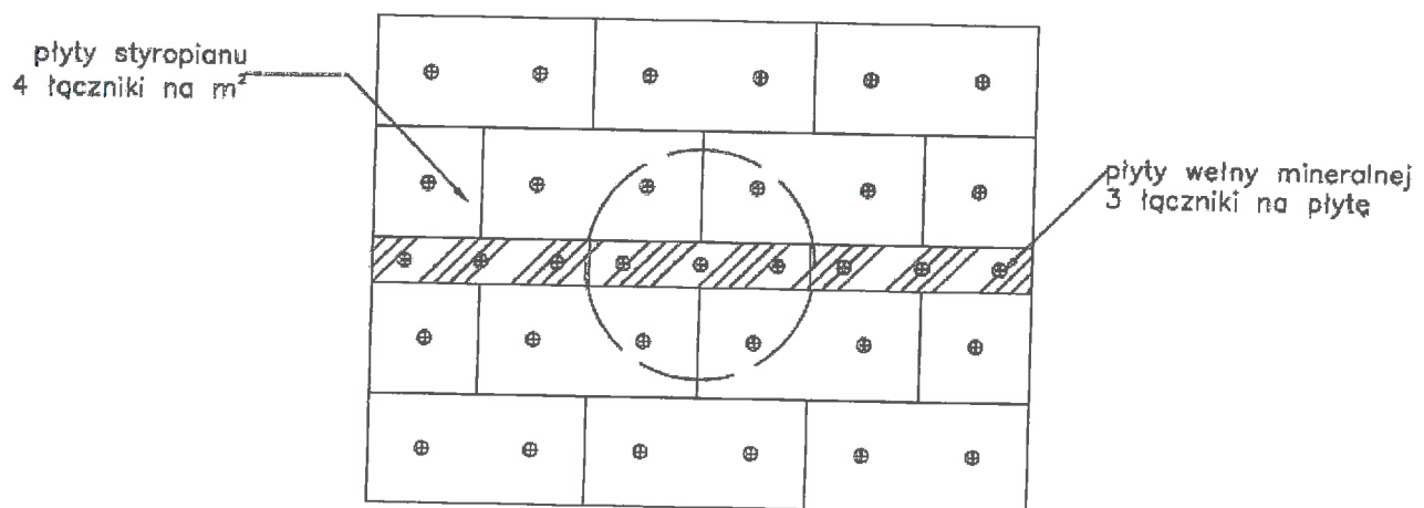
Fotografia 15. Połączenie pasa wełny mineralnej MW ze styropianem
