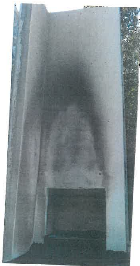
Fotografia 37. System w trakcie badania – po wygaszeniu źródła ognia
