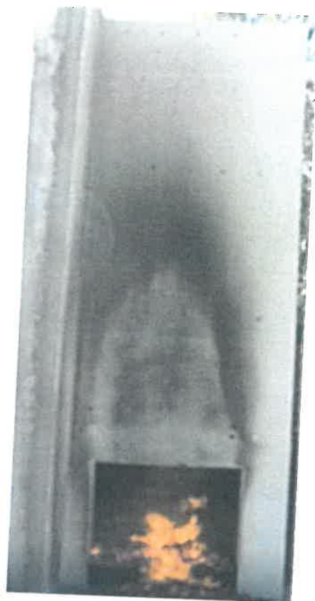
Fotografia 36. System w trakcie badania – 29 minuta badania
