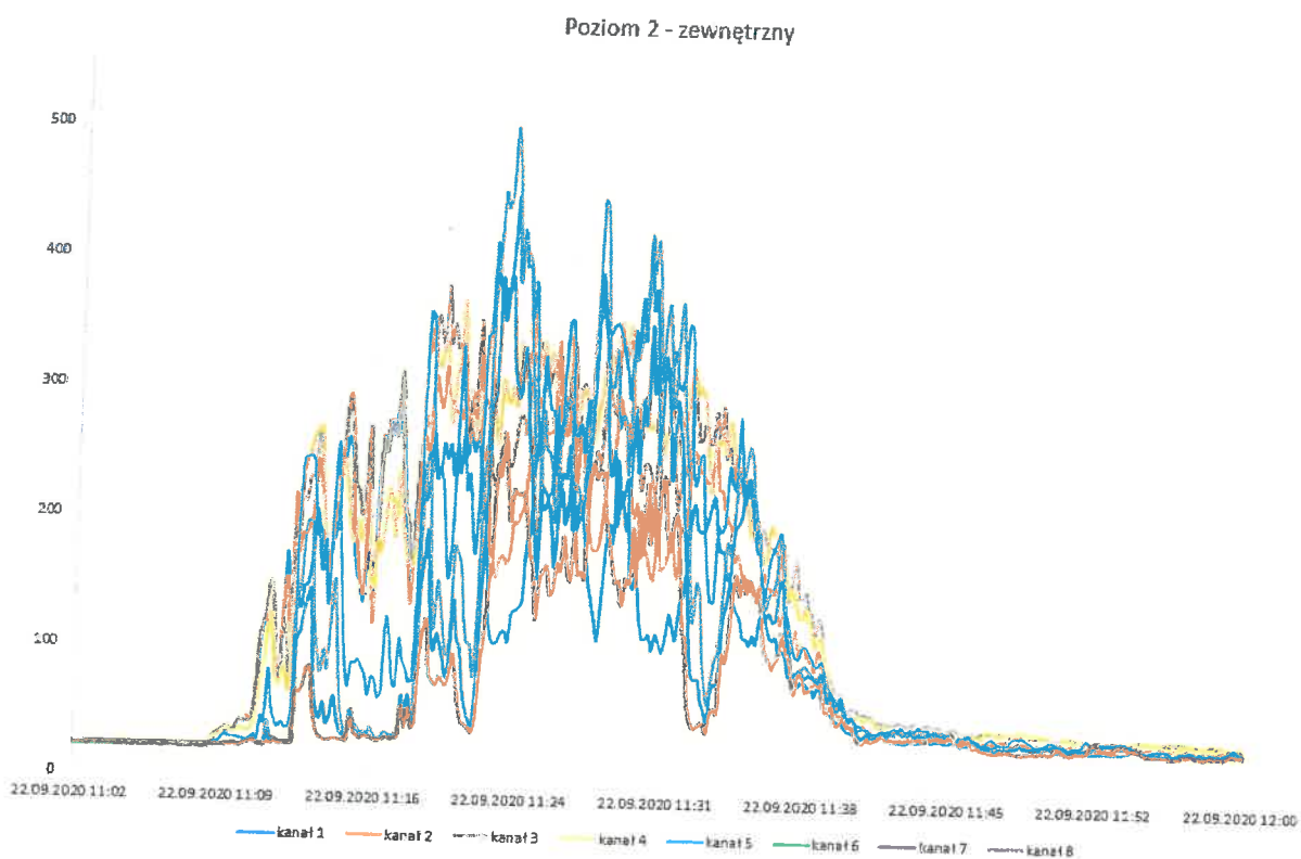
Fotografia 24. Wykres temperatury Poziom 2 - na zewnątrz
