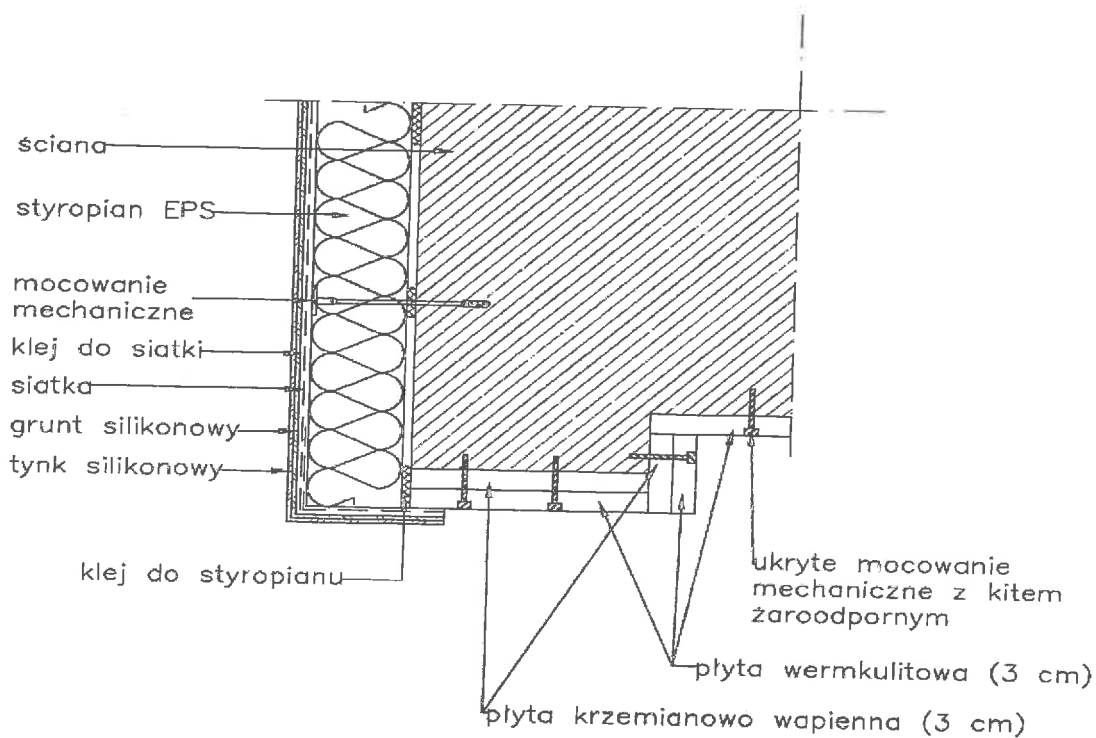
Fotografia 12. Połączenie ocieplenia z nadprożem
