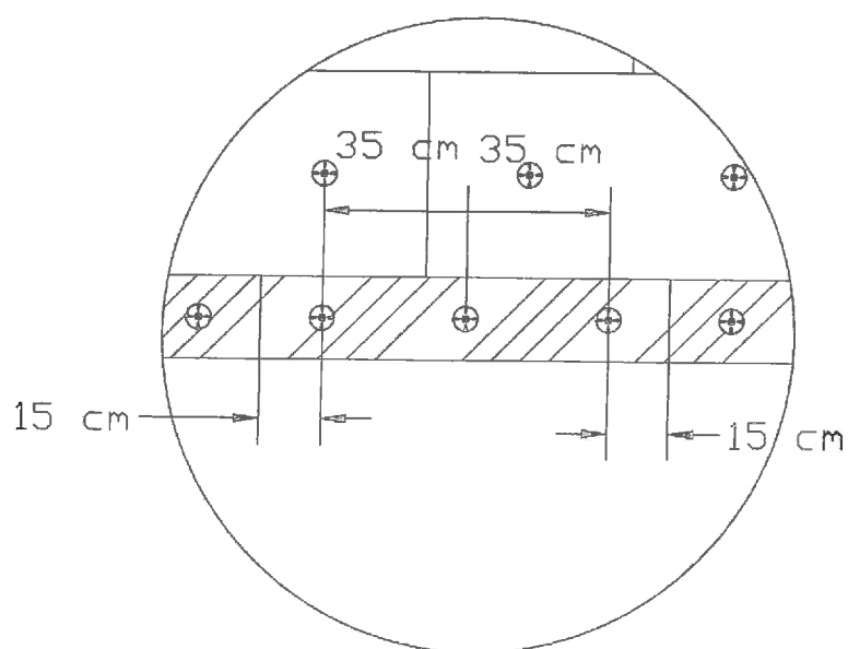
Fotografia 15. Schemat mocowania mechanicznego płyt EPS i pasa z płyt z wełny mineralnej w strefie nadproża – powiększenie
