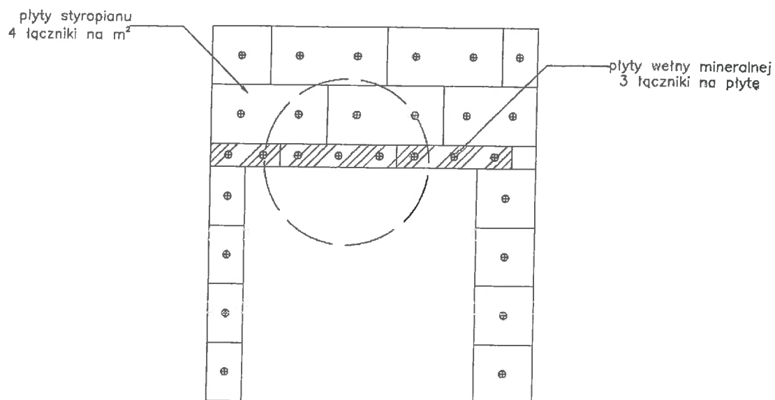
Fotografia 14. Schemat mocowania mechanicznego płyt EPS i pasa z płyt wełny mineralnej w strefie nadproża
