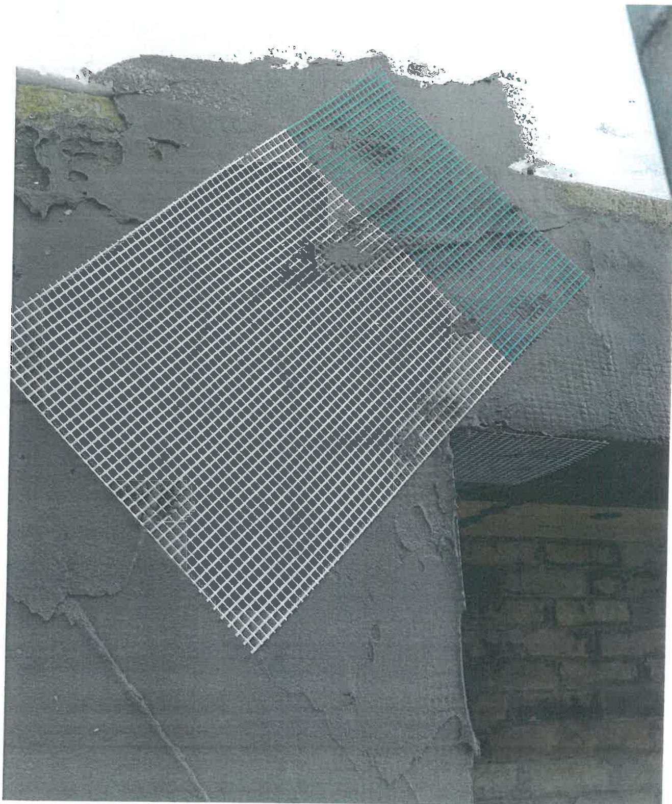
Fotografia 5. Przygotowanie systemu do badań
