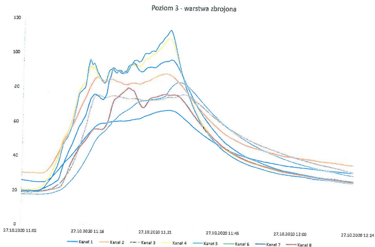
Fotografia 26. Wykres temperatury Poziom 3 – na styku warstwy zbrojącej z termoizolacją
