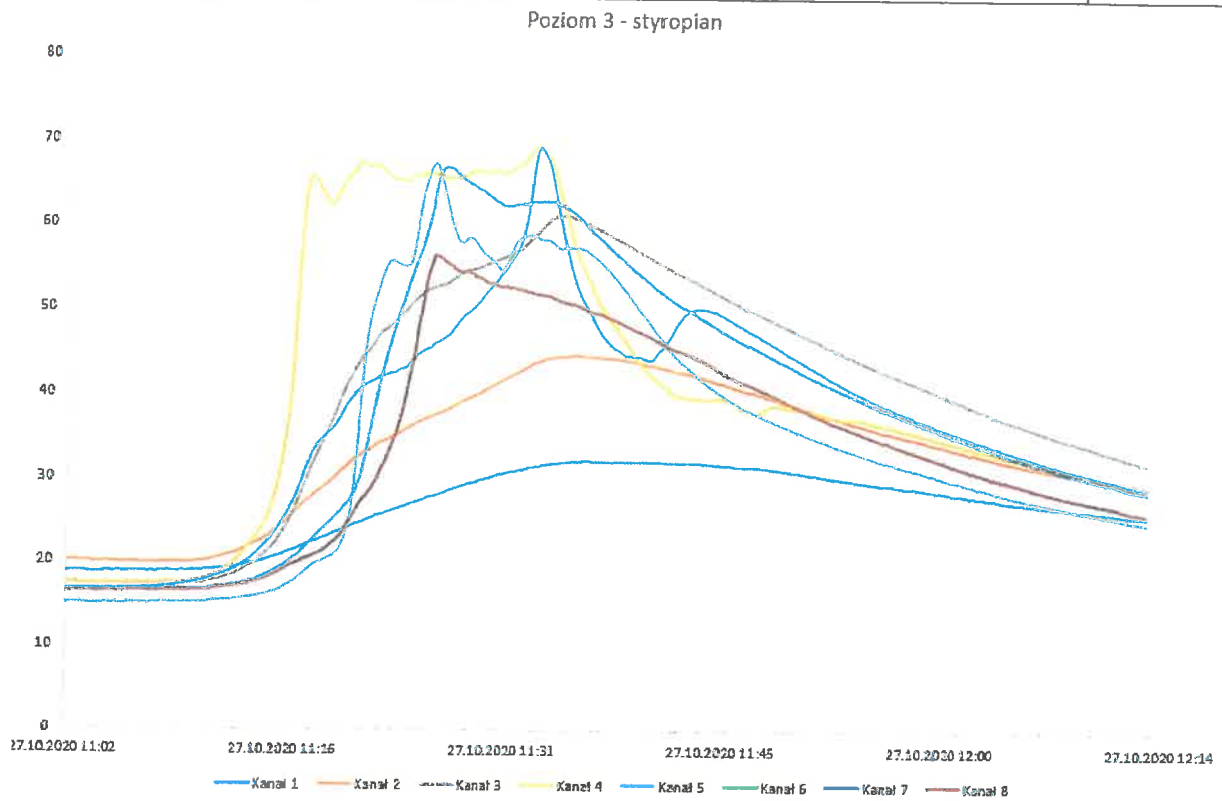
Fotografia 27. Wykres temperatury Poziom 3 – wewnątrz termoizolacji
