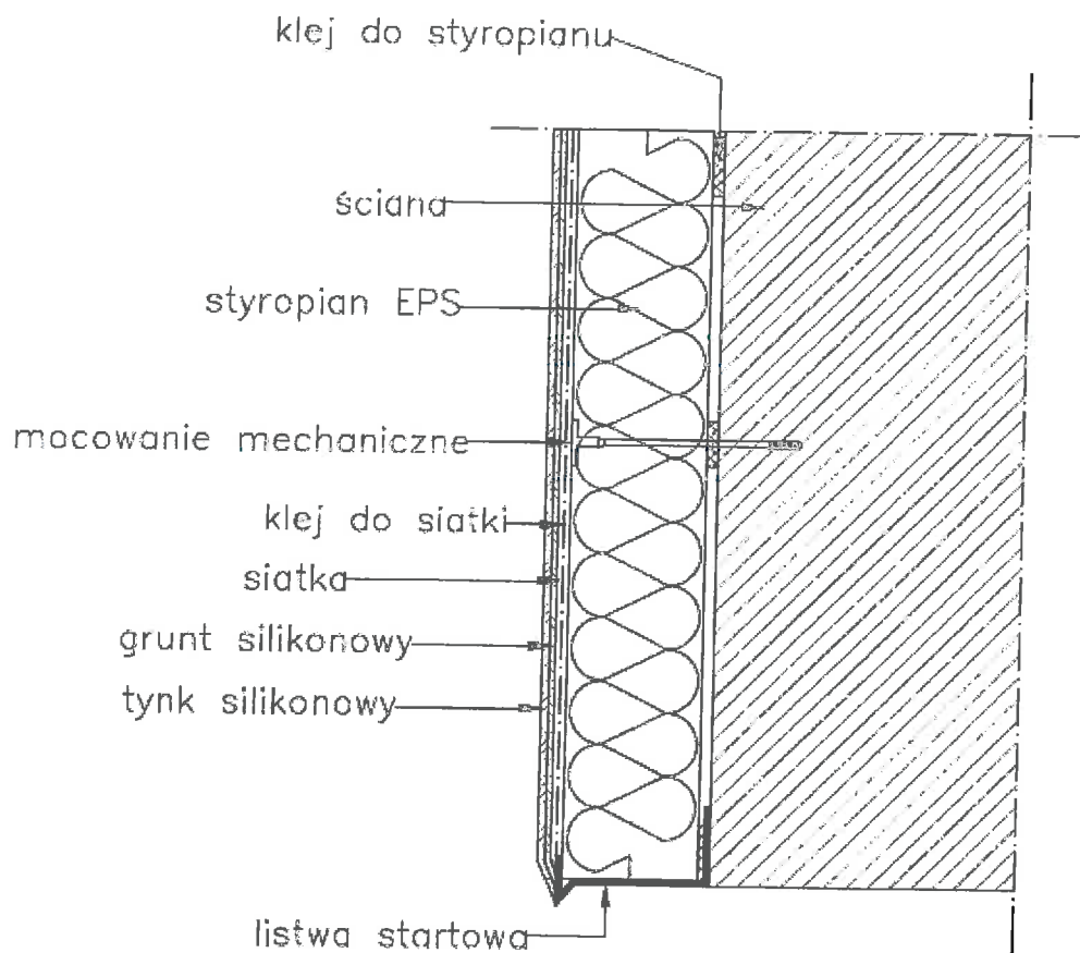
Fotografia 10. Listwa startowa
