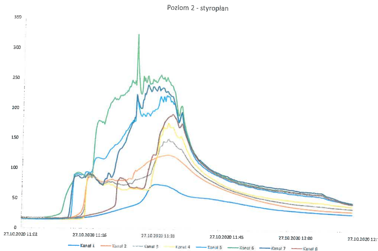
Fotografia 25. Wykres temperatury Poziom 2 – wewnątrz termoizolacji
