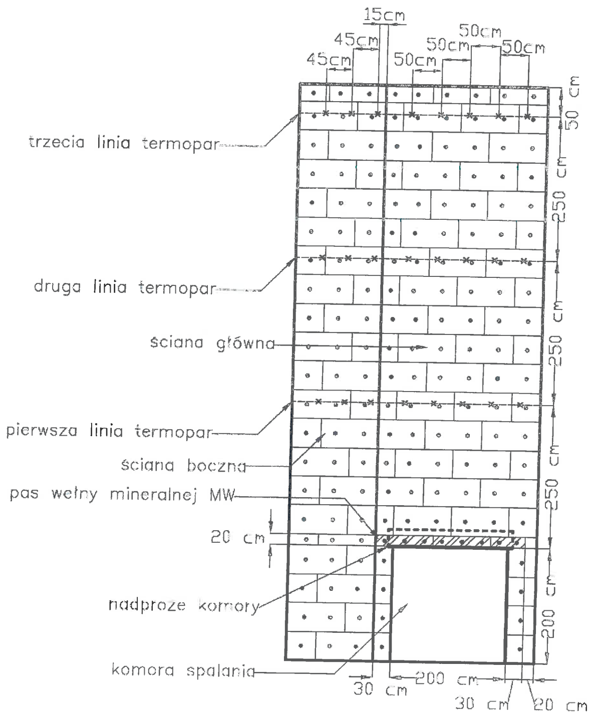
Fotografia 18. Ogólny schemat badanego systemu
